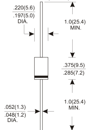
DO-201AD(DO-27)
